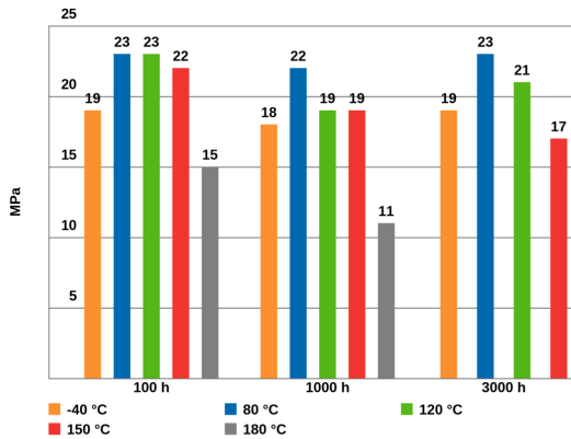
Zugscherfestigkeit nach Temperurlagerung Substrate: Al/Al, in Anlehnung an DIN EN 1465
