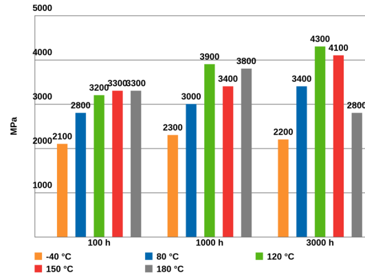
E-Modul nach Temperurlagerung, in Anlehnung an DIN EN ISO 527
