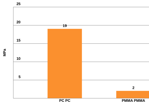
Druckscherfestigkeit auf verschiedenen Substraten, DELO-Norm 5
