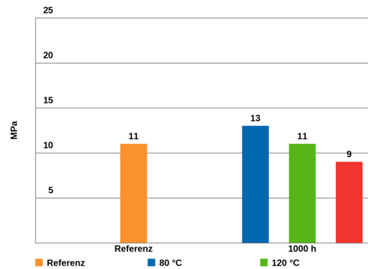
Zugscherfestigkeit nach Temperurlagerung, in Anlehnung an DIN EN 1465
