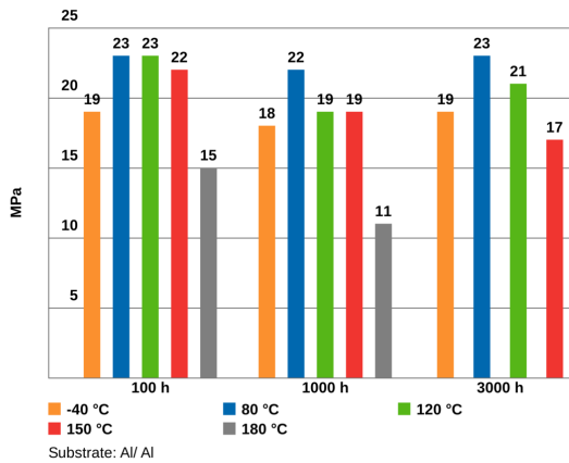
Zugscherfestigkeit nach Temperaturlagerung, basierend auf DIN EN 1465
