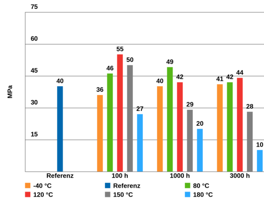
E-Modul nach Temperurlagerung Aushärtung / RT
