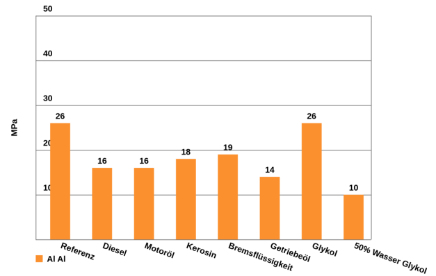
Druckscherfestigkeit nach Medienlagerung für 1000 h, DELO-Norm 5
