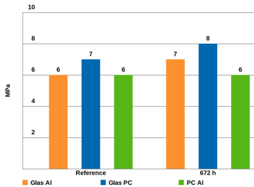
Druckscherfestigkeit nach Temperaturlagerung bei , DELO-Norm 5
