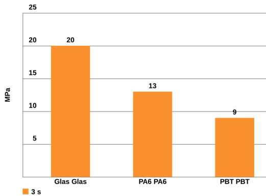
Druckscherfestigkeit nach Voraktivierung, basierend auf DELO-Norm 5
