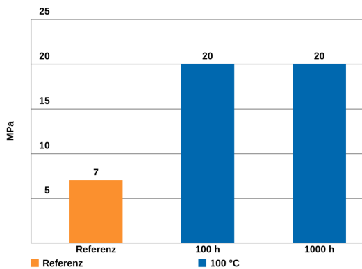
Druckscherfestigkeit nach Temperaturlagerung, basierend auf DELO-Norm 5
