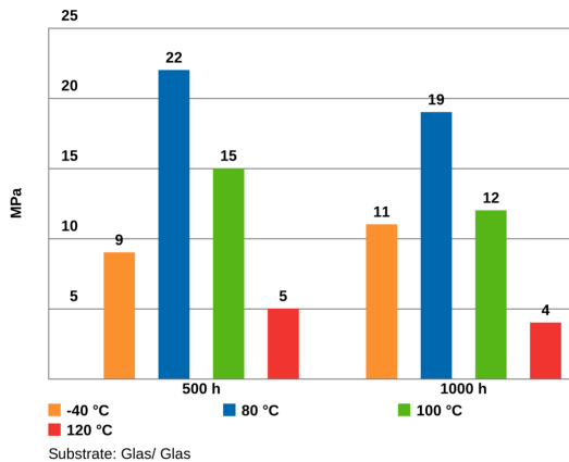
Druckscherfestigkeit nach Temperaturlagerung, basierend auf DELO-Norm 5
