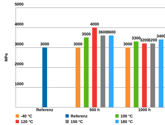
E-Modul nach Temperaturlagerung Aushärtung 60 mW/cm² 90 s /
