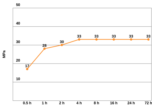
Druckscherfestigkeit für die Bestimmung des Aushärtungsprozesses Welle-Nabe-Verklebung, Substrate: Stahl Welle/Stahl Nabe, basierend auf ISO 10123
