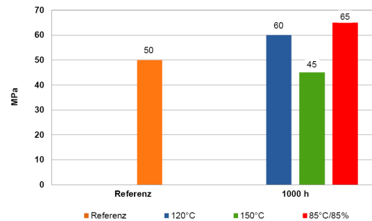
Zugfestigkeit nach Temperaturlagerung, in Anlehnung an DIN EN ISO 527 Lichtfixierung: LED 400nm, Intensity 200mW/cm², 60s
