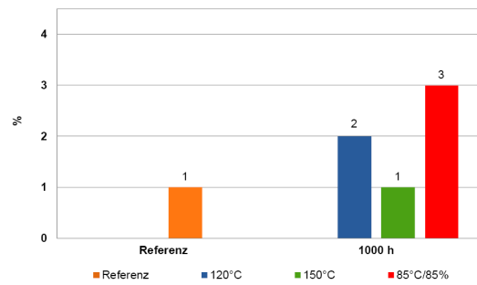
Reißdehnung nach Temperaturlagerung, in Anlehnung an DIN EN ISO 527 Lichtfixierung: LED 400nm, Intensity 200mW/cm², 60s
