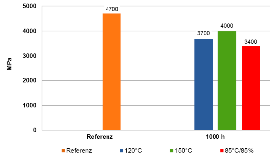
E-Modul nach Temperaturlagerung, in Anlehnung an DIN EN ISO 527 Lichtfixierung: LED 400nm, Intensity 200mW/cm², 60s
