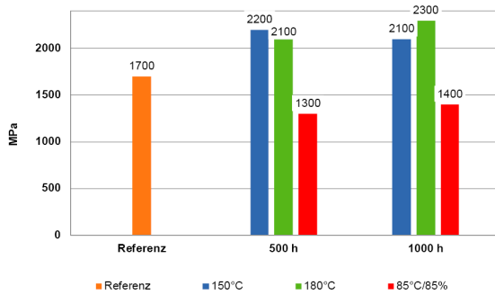
E-Modul nach Temperaturlagerung, in Anlehnung an DIN EN ISO 527 Aushärtung: 7d RT
