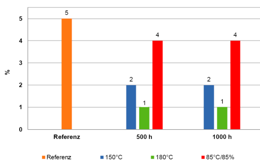
Reißdehnung nach Temperaturlagerung, in Anlehnung an DIN EN ISO 527 Aushärtung: 7d RT
