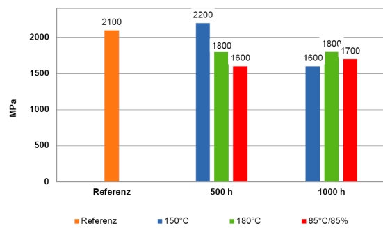
E-Modul nach Temperaturlagerung, in Anlehnung an DIN EN ISO 527 Aushärtung: 1h +80°C
