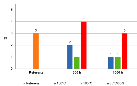
Reißdehnung nach Temperaturlagerung, in Anlehnung an DIN EN ISO 527 Aushärtung: 1h +80°C
