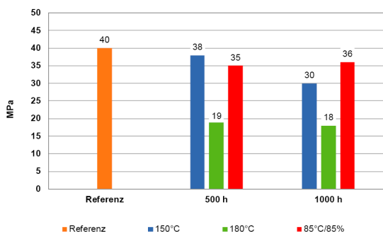
Zugfestigkeit nach Temperaturlagerung, in Anlehnung an DIN EN ISO 527 Aushärtung: 7d RT
