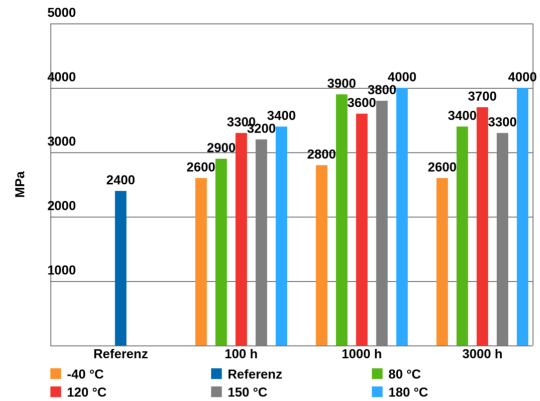
E-Modul nach Temperaturlagerung, in Anlehnung an DIN EN ISO 527
